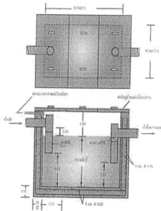
บ่อตกไขมันแบบสร้างในที่สำหรับอาคารขนาดใหญ่
